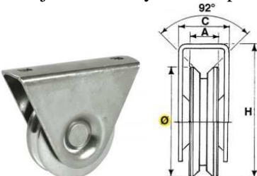
Koło jezdne 1-łożyskowe z podporą górną V
