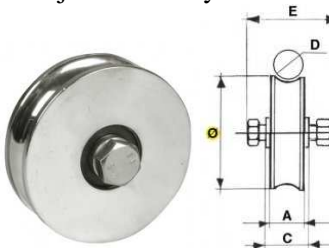
Koło jezdne 2-łożyskowe U
