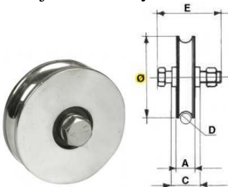
Koło jezdne 1-łożyskowe U
