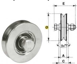
Koło jezdne 1-łożyskowe V
