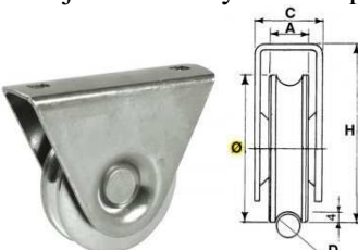
Koło jezdne 1-łożyskowe z podporą górną U
